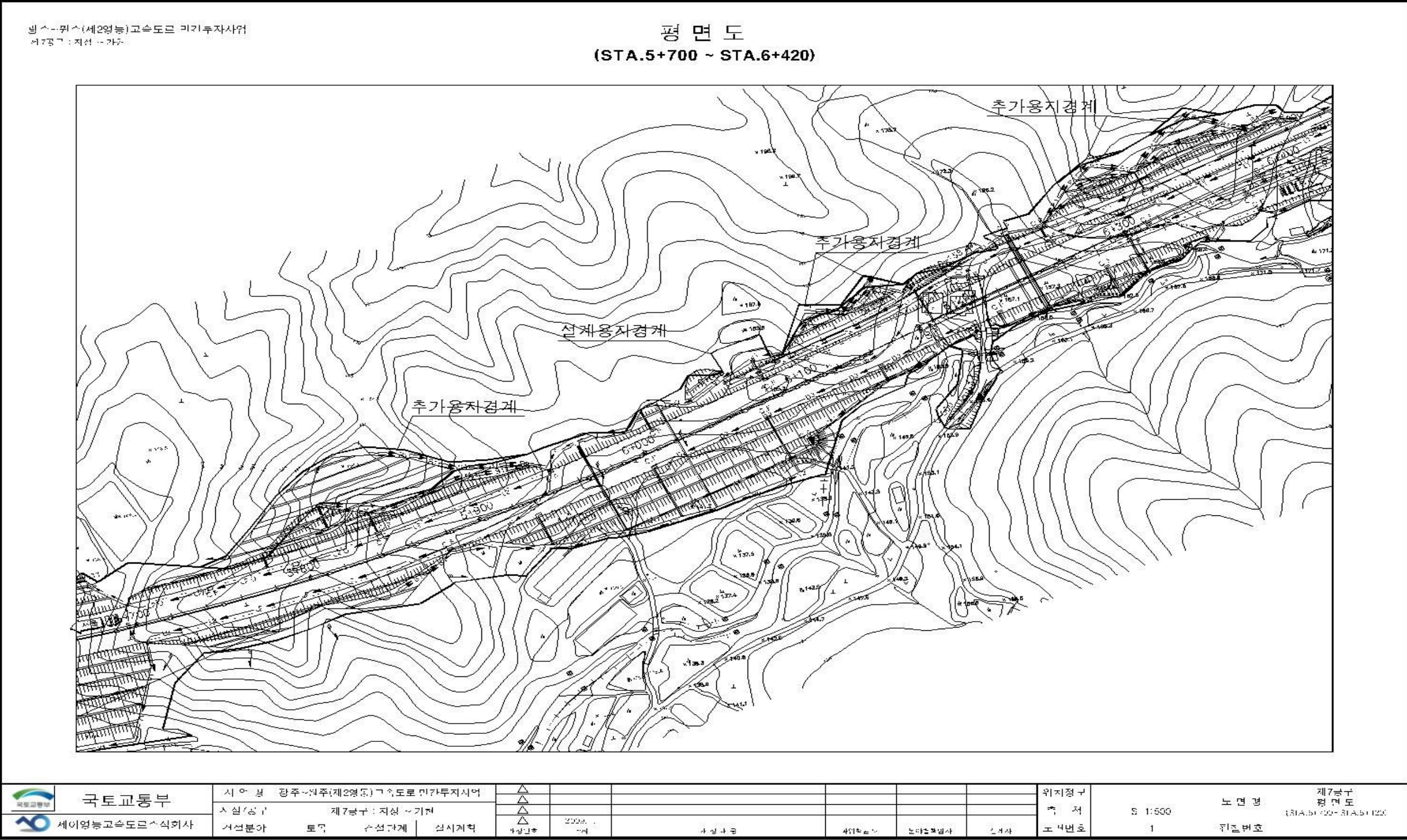
【그림 1.3-1】 평면도
