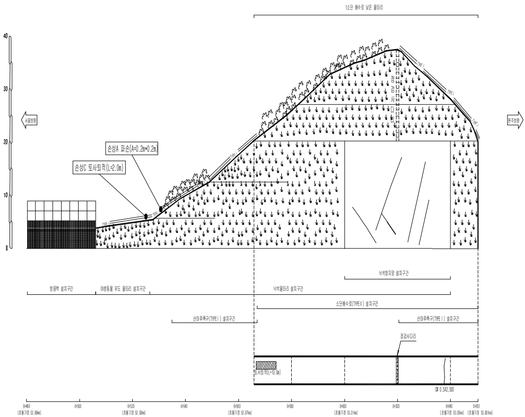
절토사면 STA.6+480~6+651/초월기점 52.89~53.061km (서울방향)
