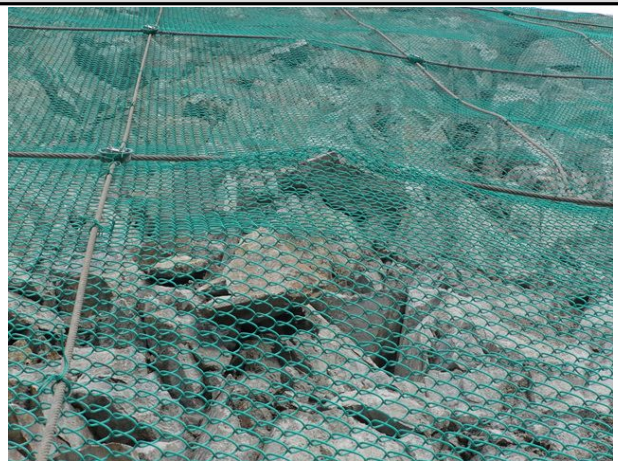
53.03K 1단 낙석방지망 내부 이완암 및 뜬돌
